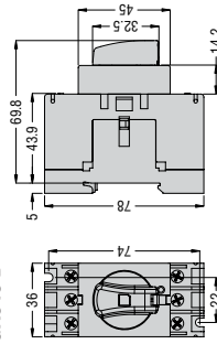
GA016 A...GA040 A GA040 D
